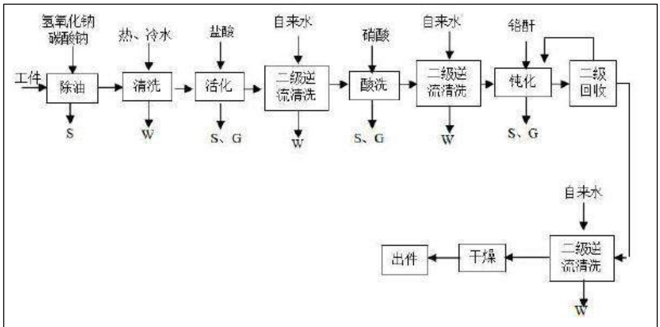
图 1-1 工艺流程及产污节点图
