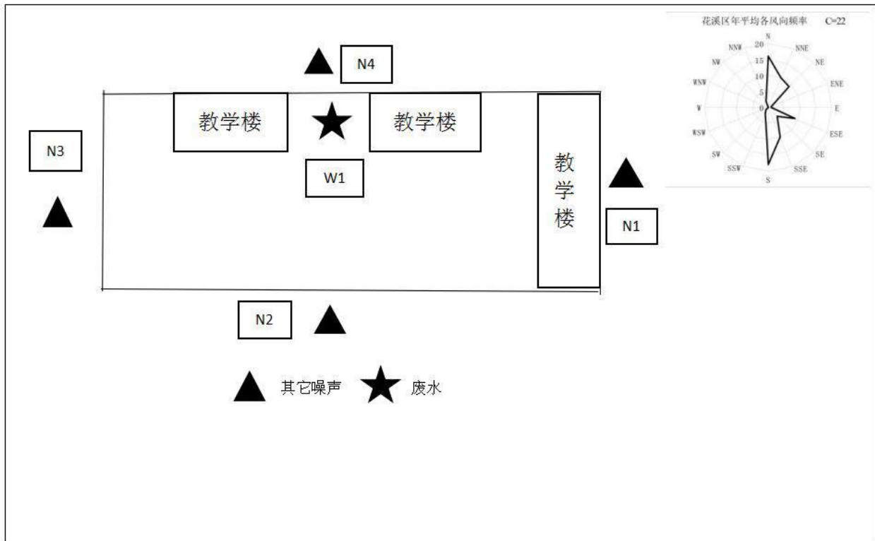
采样布点图
